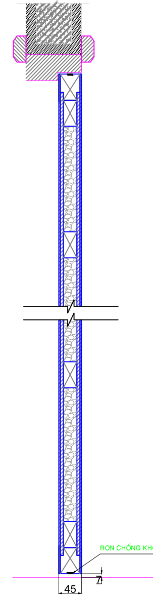
MẶT CẮT 1-2 TL : 1/5
