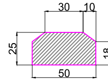
CT : CHỈ KHUNG BAO TL : 1/2
