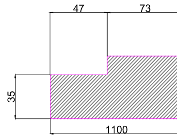
CT : KHUNG BAO TL : 1/2
