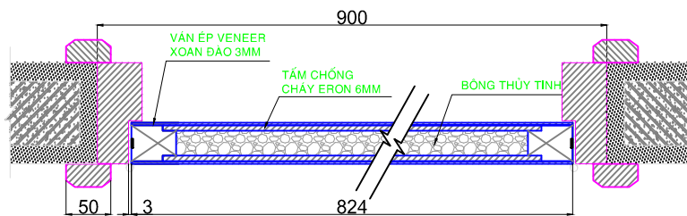
MẶT CẮT 1-1 TL : 1/5
